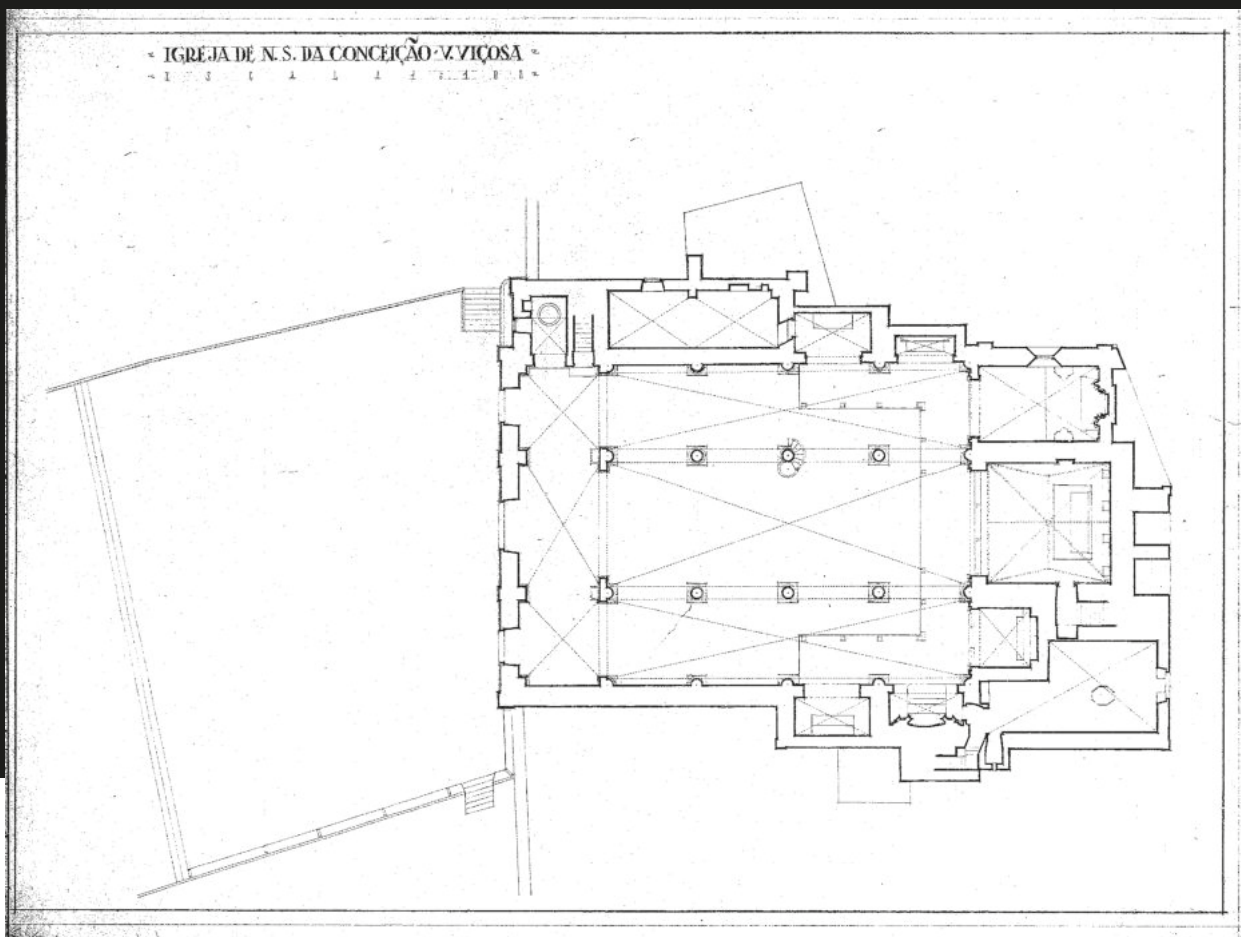
Fig. 54 – Vila Viçosa, Igreja de Nossa Senhora da Conceição, planta geral (DGPC: SIPA DES.00001140, s.a., s. d.) e, em baixo, nave central. Foto FL, 2018.
