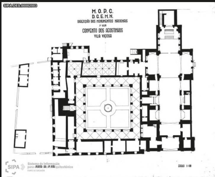
Fig. 74 – Igreja de Nossa Senhora da Graça e Convento dos Agostinhos. Planta do piso térreo (DGPC: SIPA DES.00002003, s.a., s.d.).
