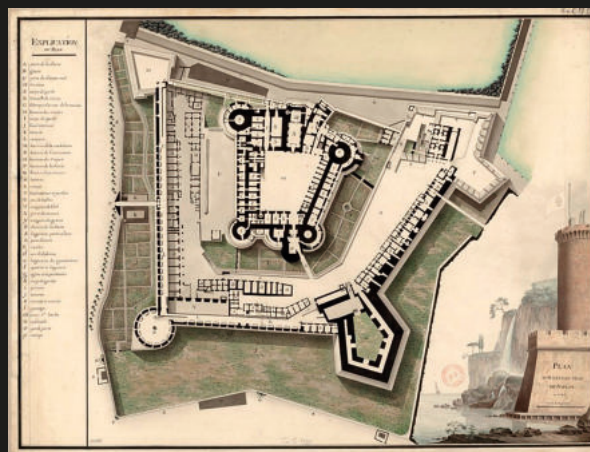
Fig. 26 – Napóles. Planta do Castel-Nuovo de 1787. Ver a analogia relativamente a Vila Viçosa, nomeadamente a adição à anterior fortificação (1497) do baluarte Vauban (1633-1707), reportado ao arquiteto e engenheiro militar francês.
