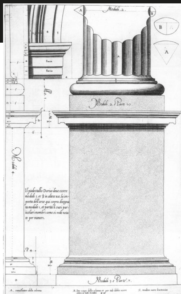
Fig. 60 – G: B. Vignola, Regola delle cinque ordine d'Architettura , Roma, 1562 (1.a ed.), intercolúnio com pedestal e fuste estriado da ordem dórica.
